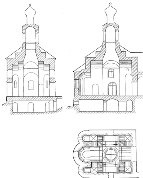
Ил. 7. Храм Рождества Богородицы в Городне. Поперечный и продольный разрезы и план. Обмер Б. Л. Альтшуллера. Опубликовано: Галашевич А. А., Колпакова Г. С. Храм Рождества Богородицы в Городне на Волге. М., 2004. С. 53.
